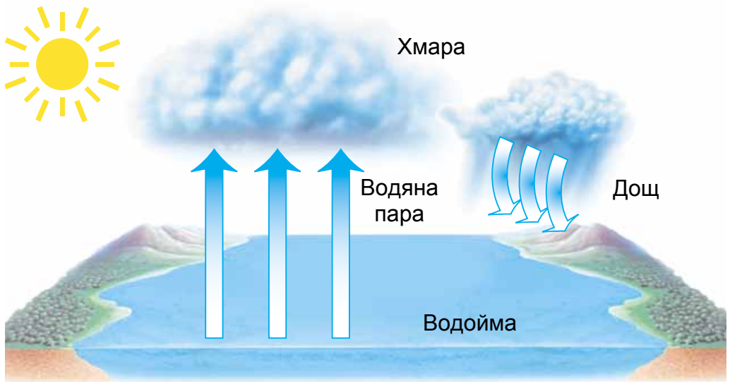
Мал. 6. Утворення хмари
